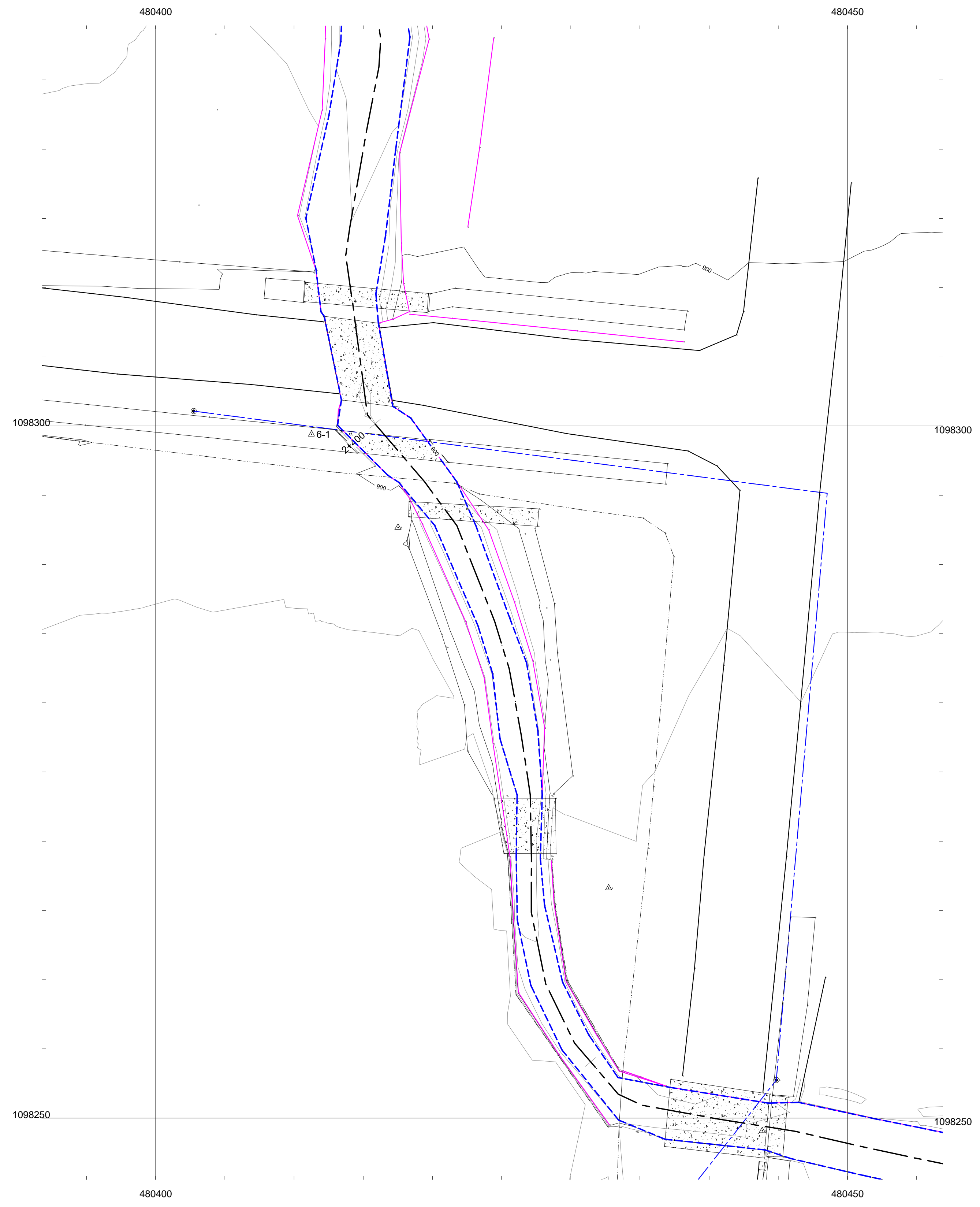
PUENTE 8 y 9 ESCALA HORIZONTAL 1:200
