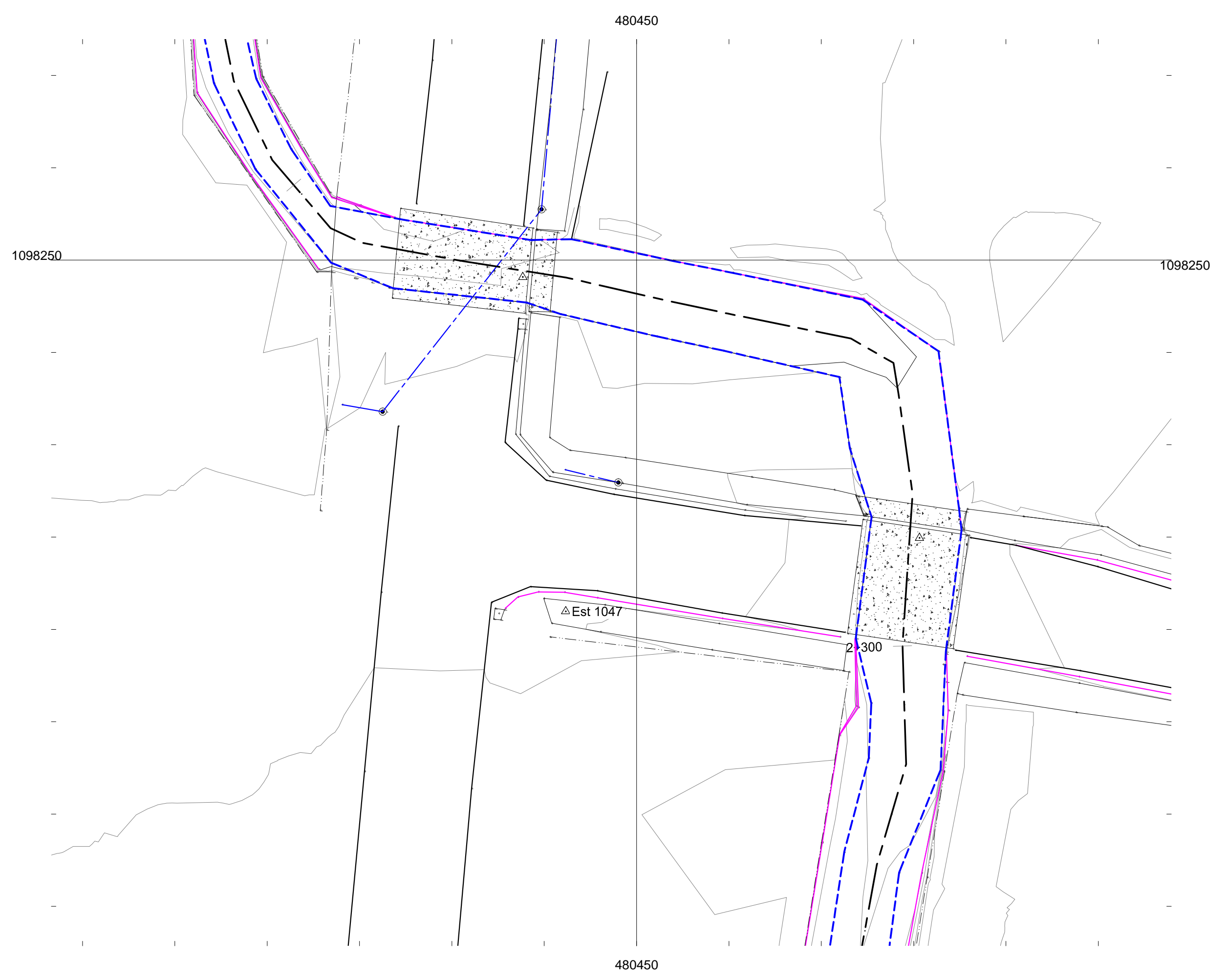
PUENTE 6 Y 7 ESCALA HORIZONTAL 1:200
