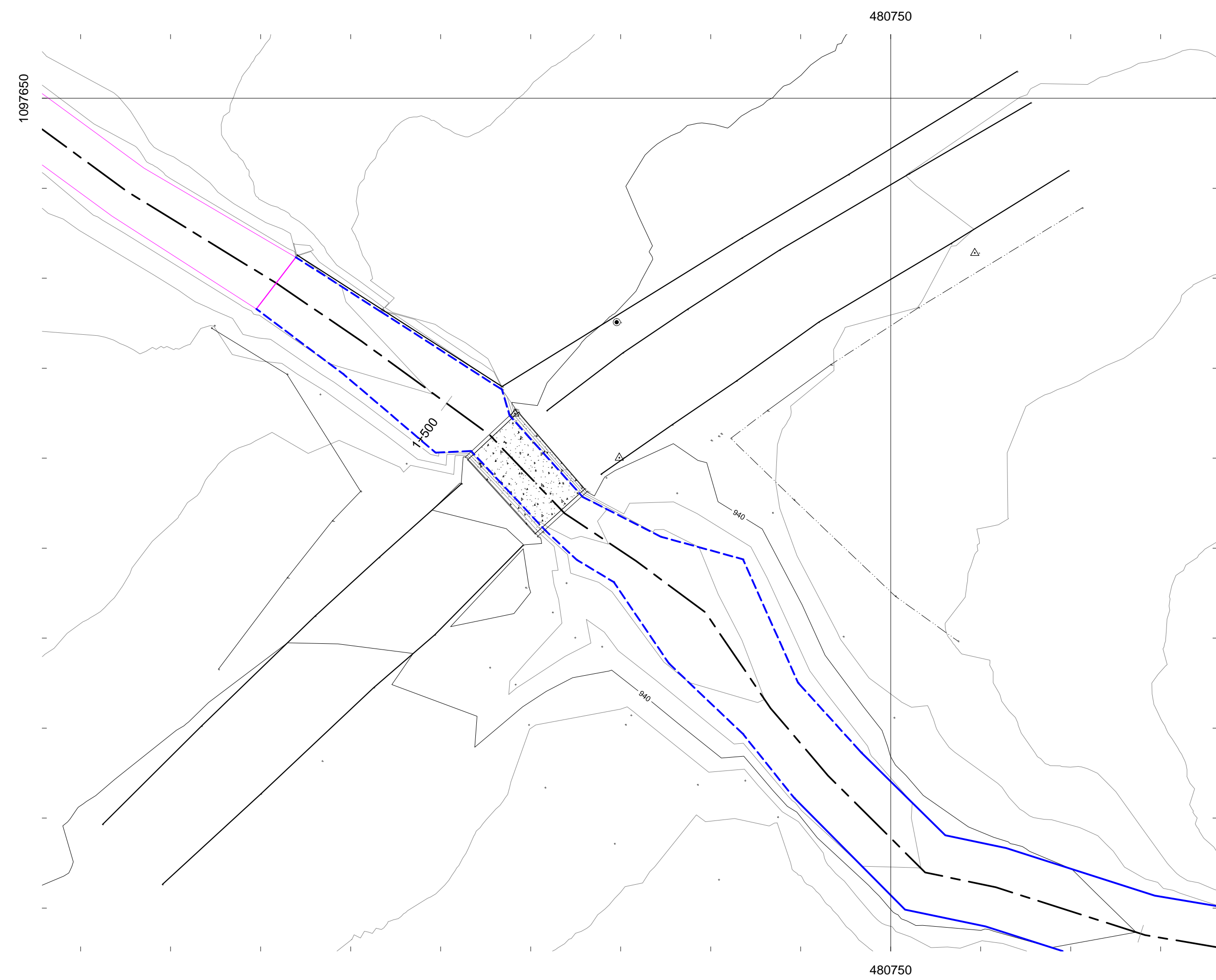
PUENTE 3 ESCALA HORIZONTAL 1:200
