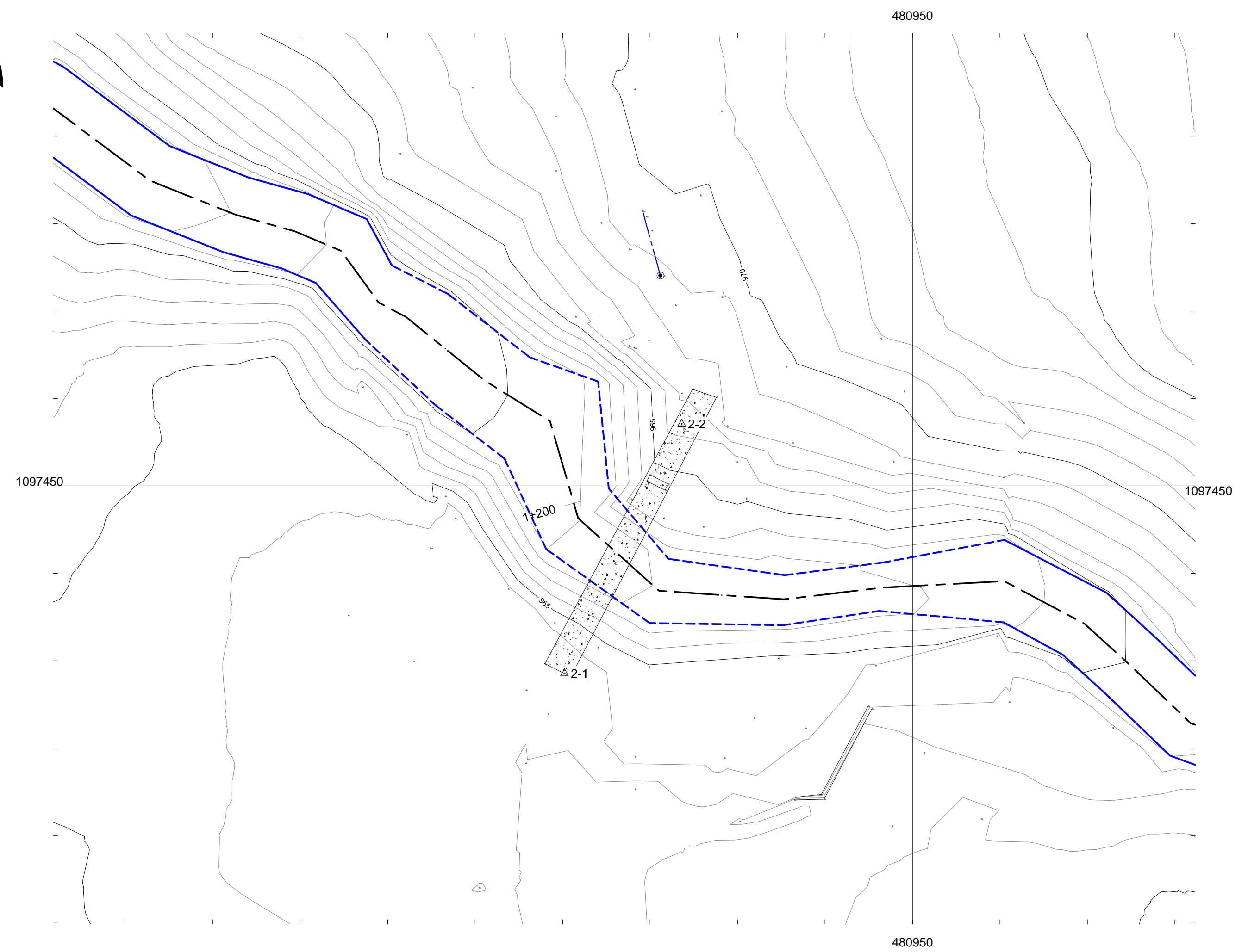
PUENTE 2 ESCALA HORIZONTAL 1:200
