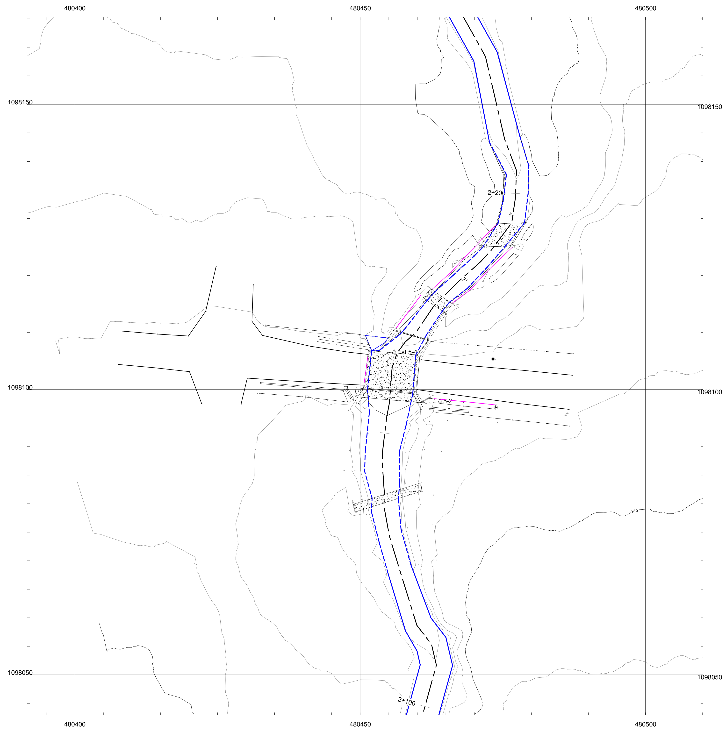
PUENTE 5 ESCALA HORIZONTAL 1:200
