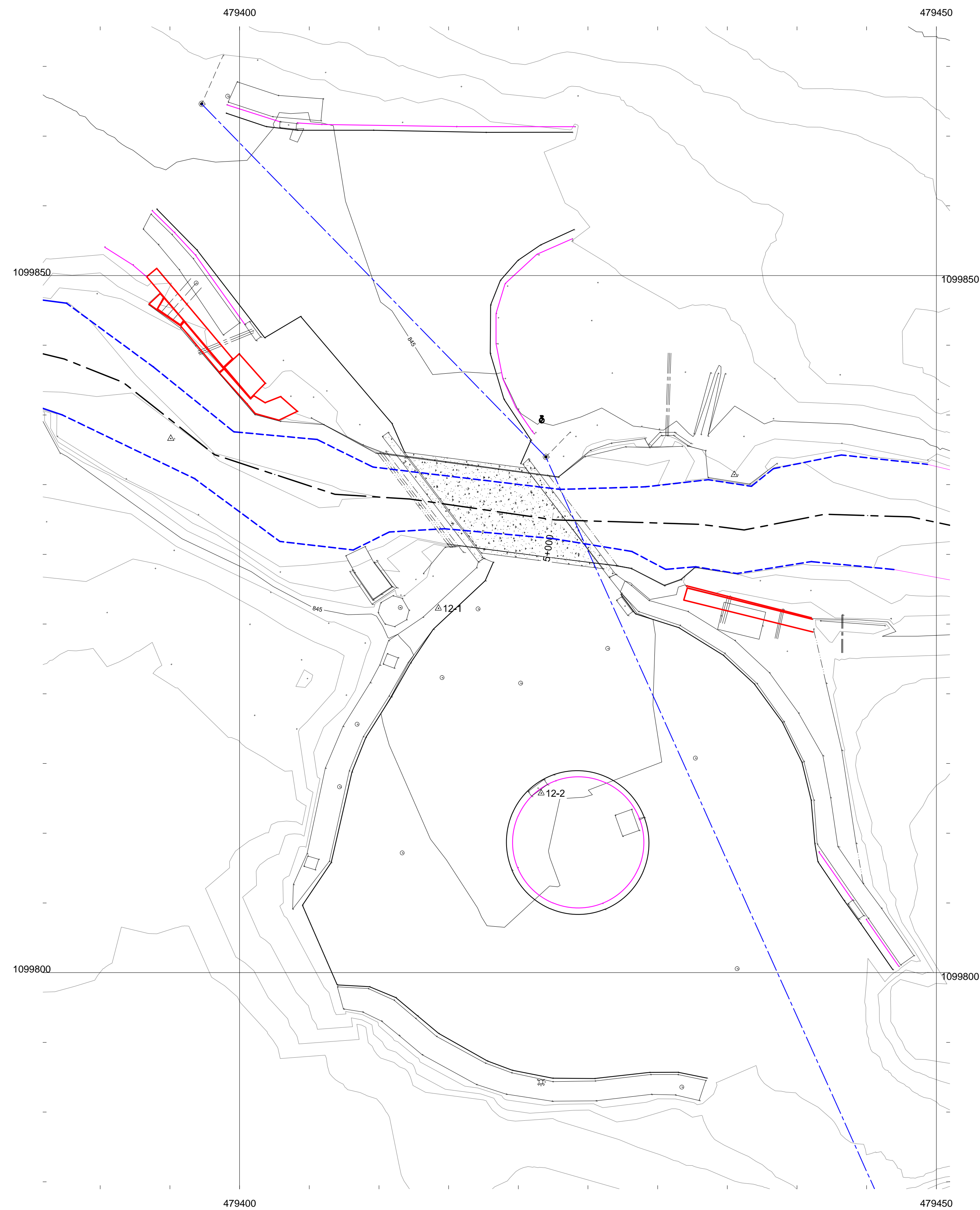
PUENTE 18 ESCALA HORIZONTAL 1:200
