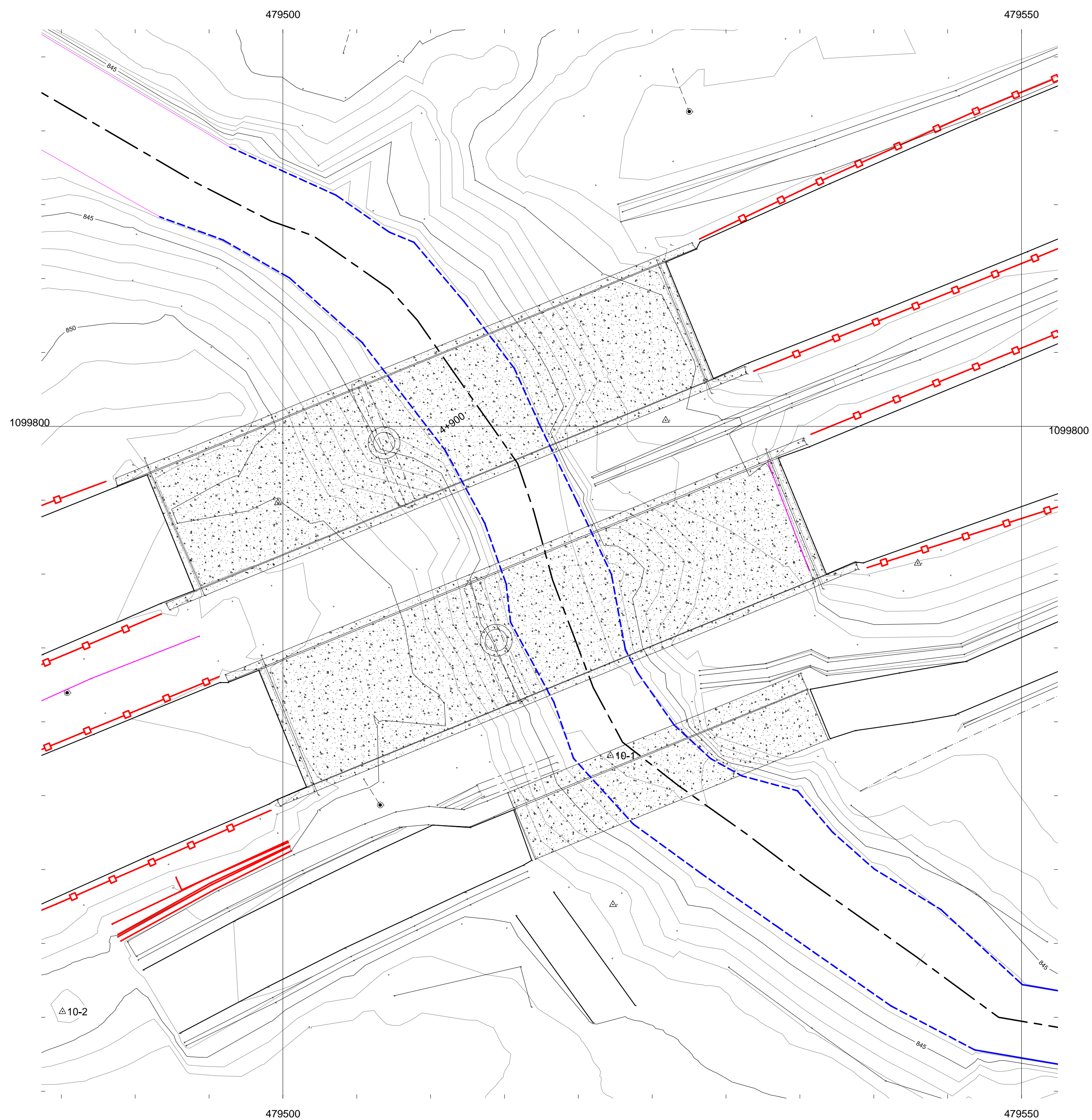
PUENTE 16 y 17 ESCALA HORIZONTAL 1:200
