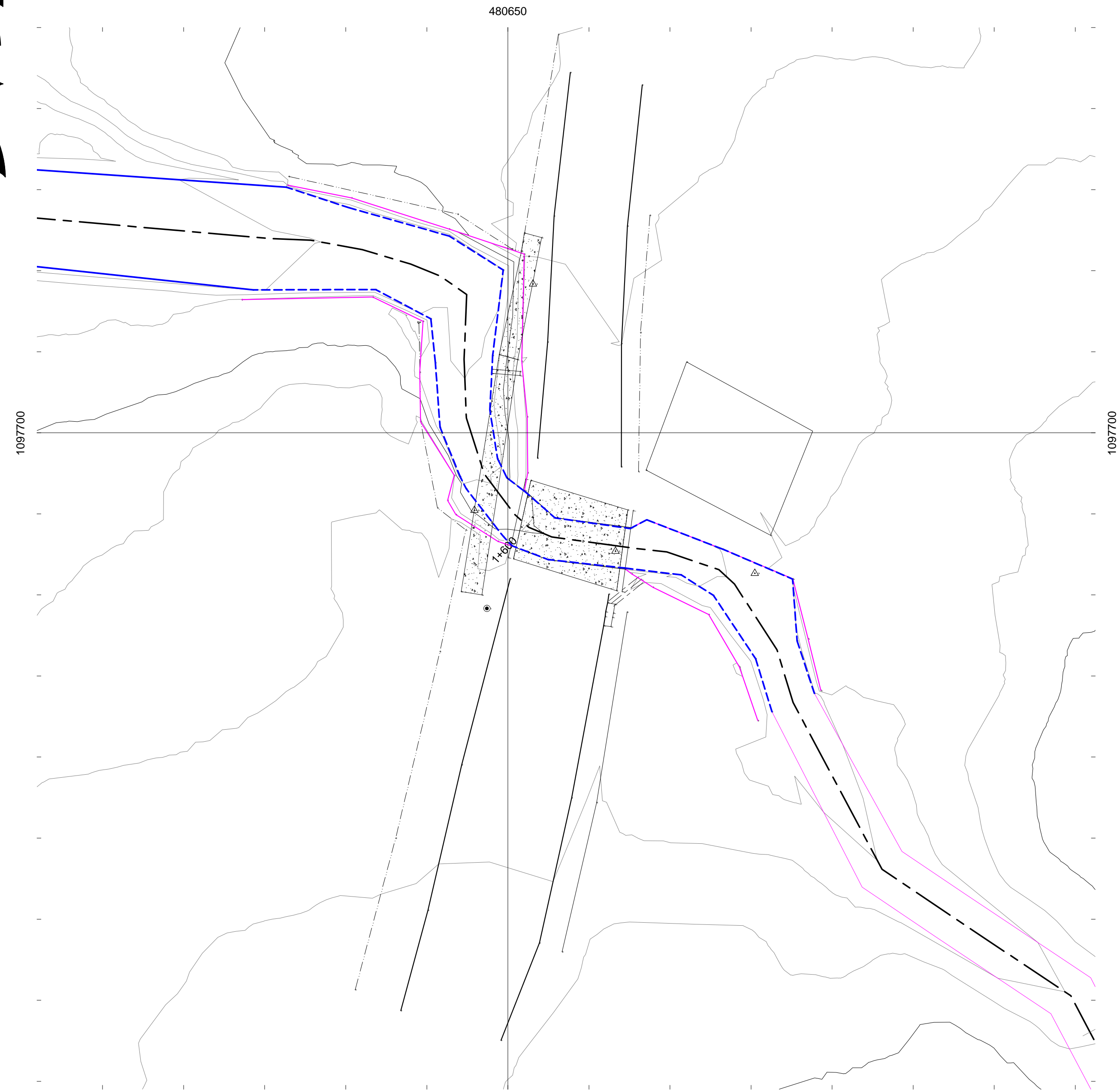
PUENTE 4 ESCALA HORIZONTAL 1:200
